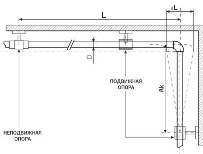
Рисунок 2. Г-образный компенсатор
