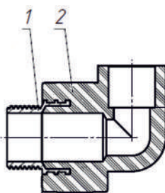
Рисунок 11. Комбинированный фитинг
