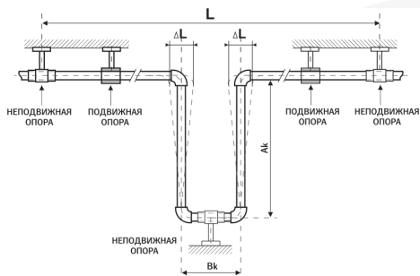
Рисунок 3. П-образный компенсатор
